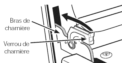
Remonter les verrous pour les enclencher
